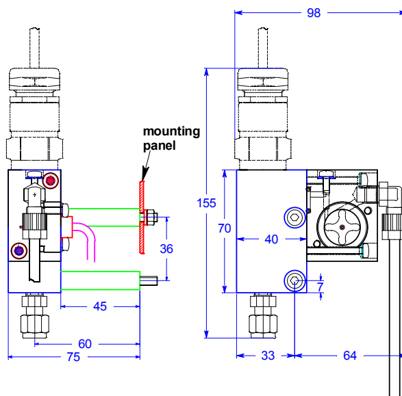
(Výkres: Q-flow SS316L 70)
